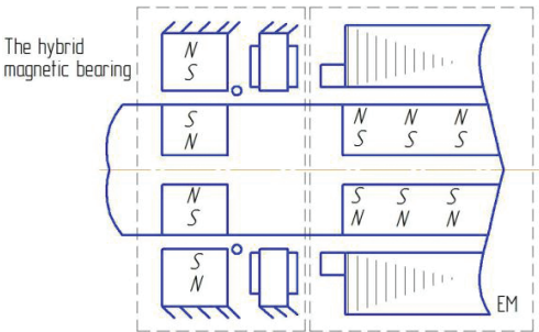
Figure 4. HMB where AMB and MB PM used separately.
